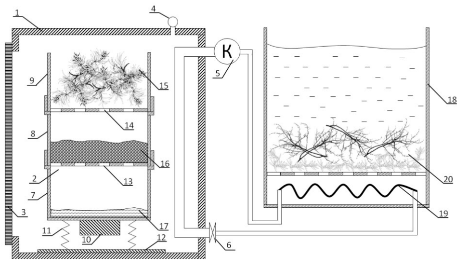
Рис. 1. Схема установки переработки плодоносящих веток облепихи на основе принципа теплового насоса
